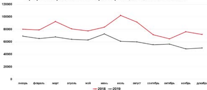
График потребления электроэнергии (kWh) 2018-2019гг.
